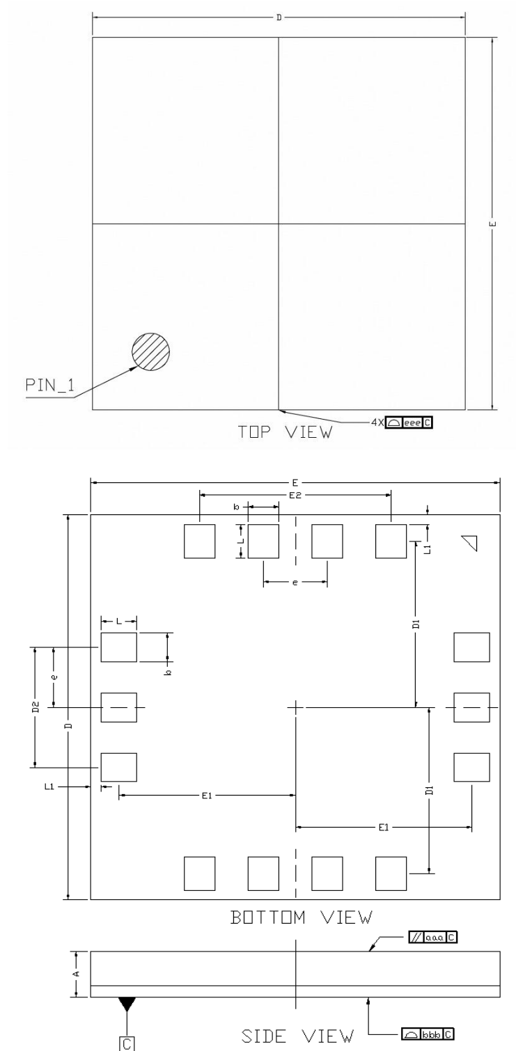
图 3.1 芯片尺寸
