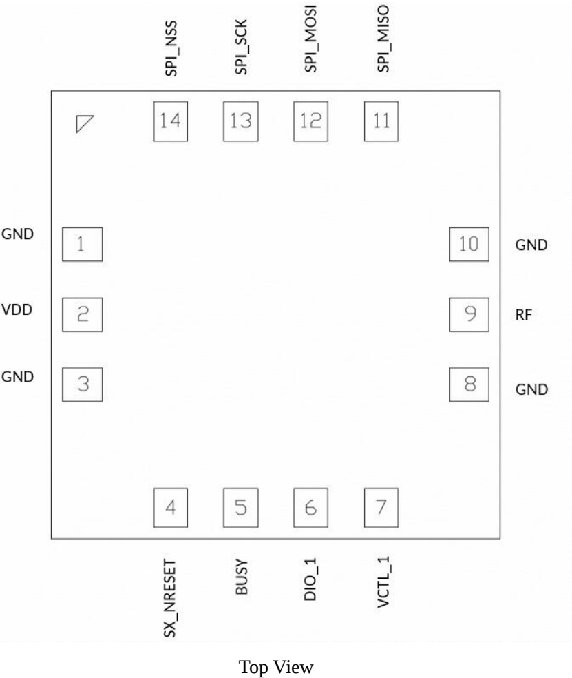
图 1.1 引脚分布图
