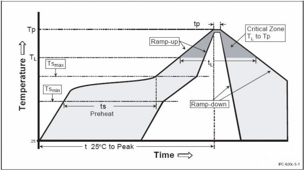
图 4.1 推荐温度曲线
